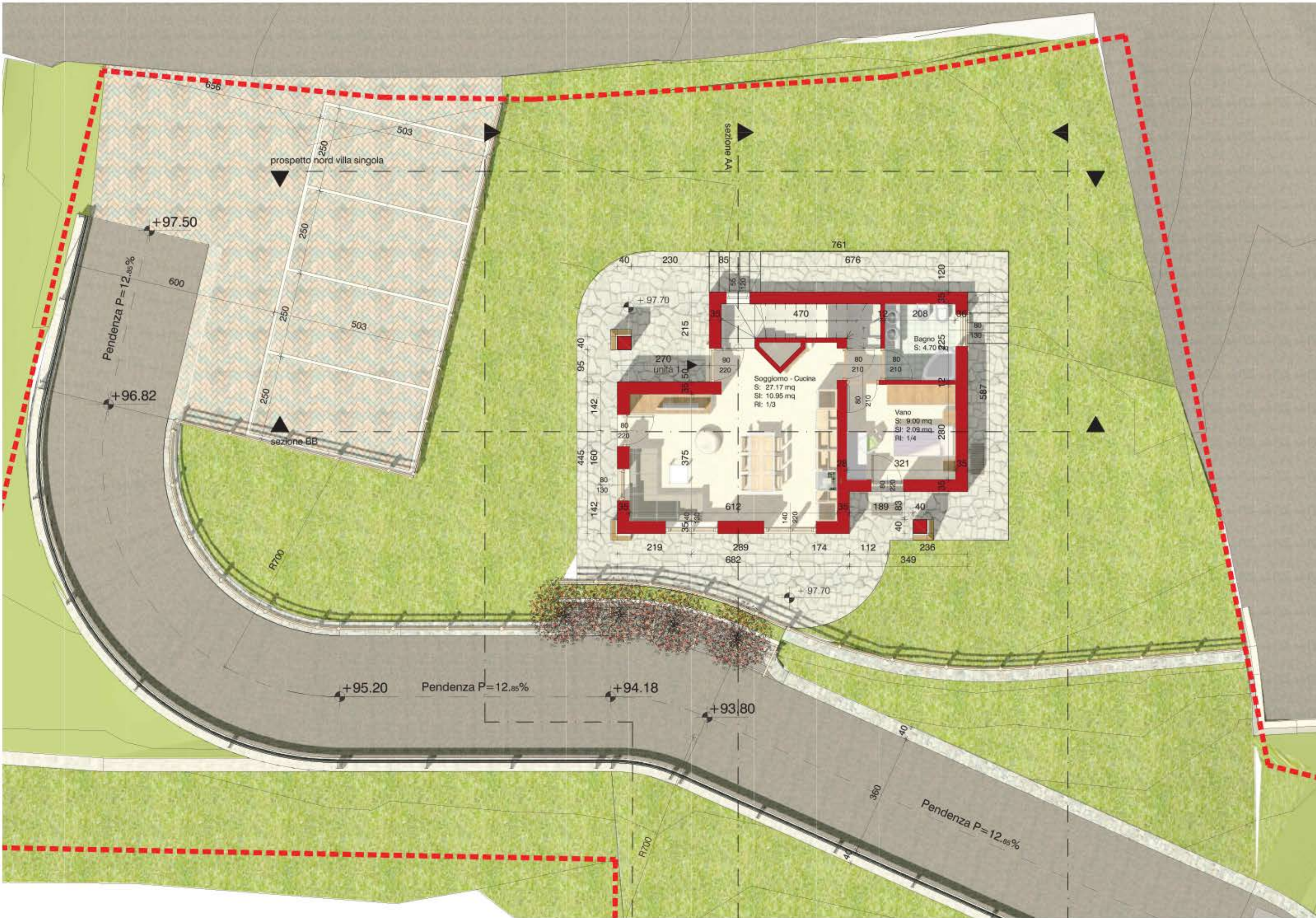
Pianta Piano Terra villa singola unità 1
