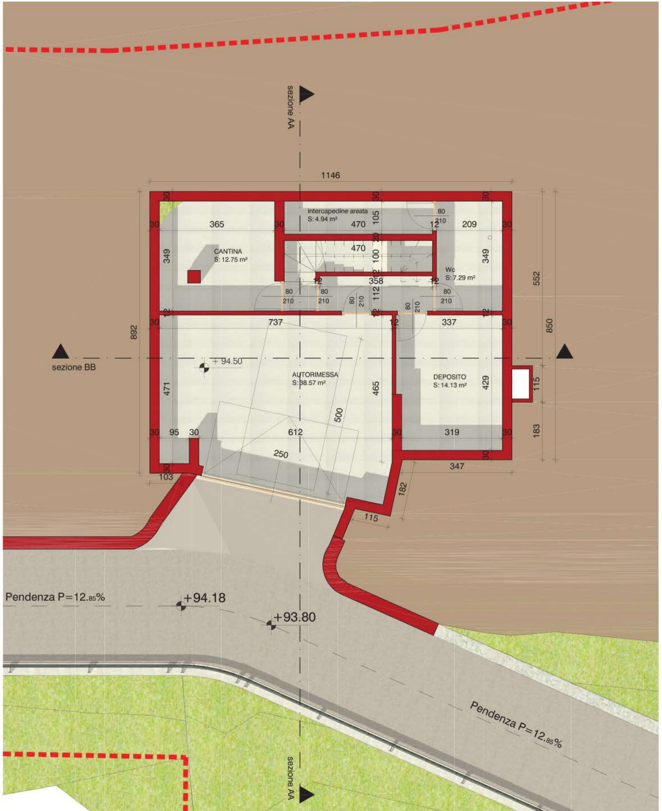
Pianta Piano Interrato villa singola unità 1
