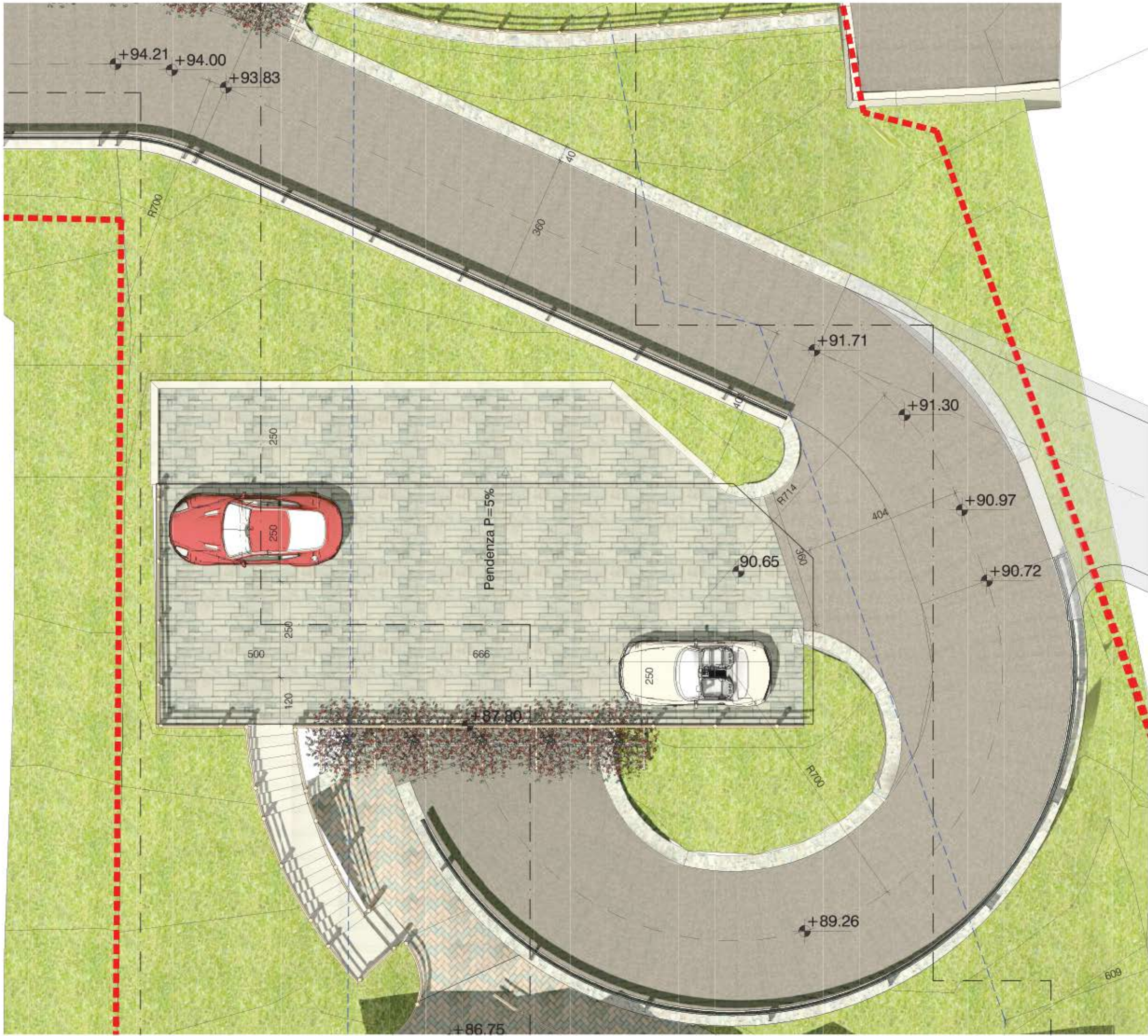
Pianta parcheggi esterni
